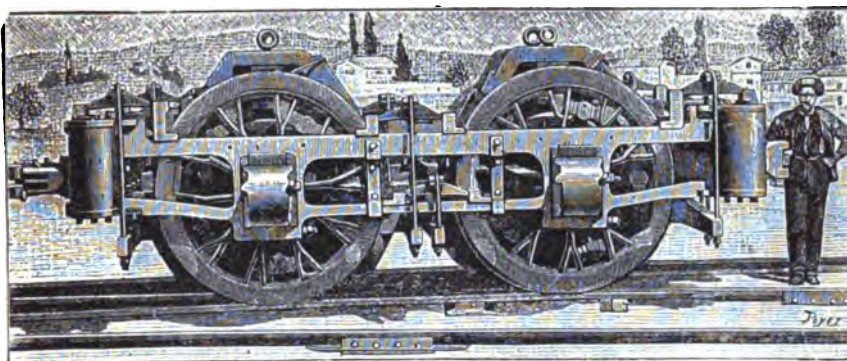
1. Телѣжка электрическаго локомотива.
